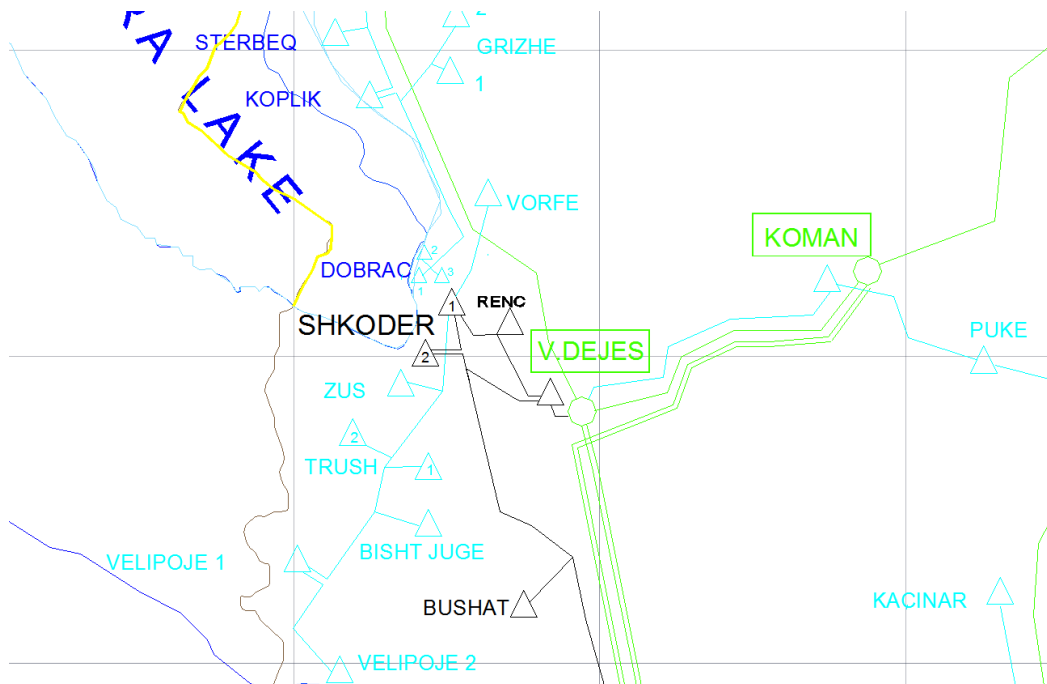
Fig. 68: Rrjeti energjetik rajonal
