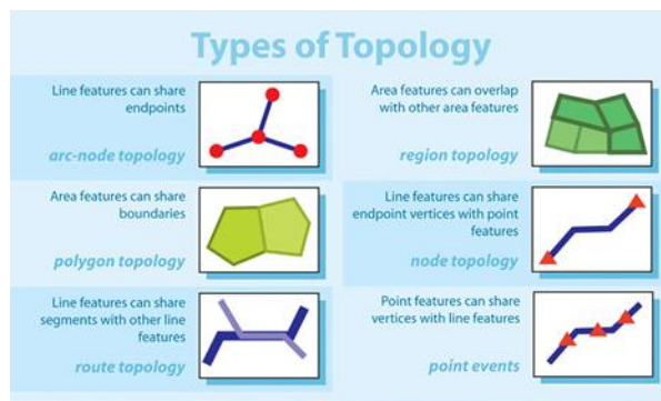
Fig. 78: Paraqitje skematike e tipeve të topologjisë
