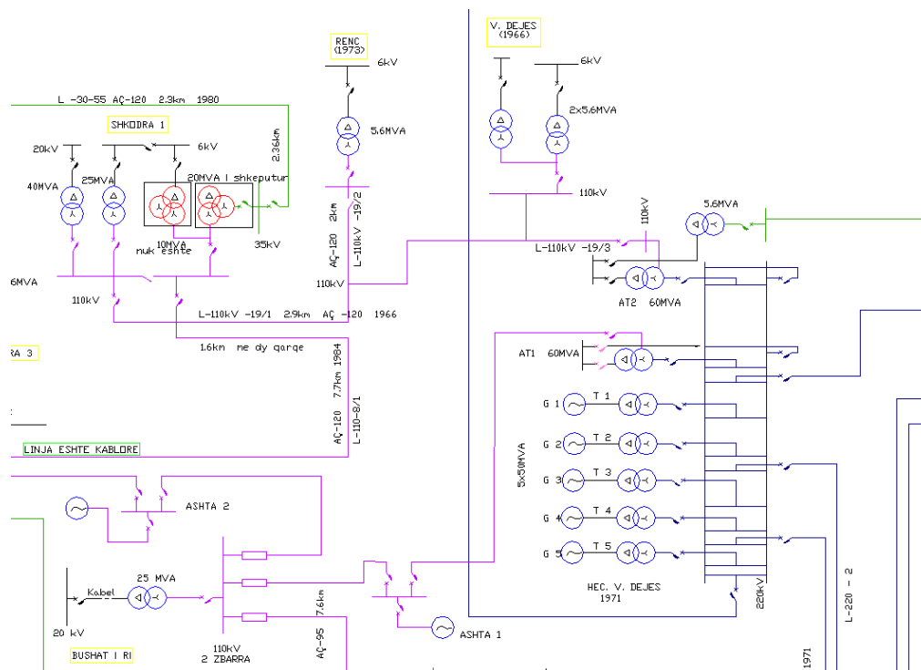
Fig. 69: Skema e rrjetit prodhues te energjise elektrike, rajoni V. Dejes
